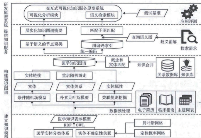
图 38 生物医药
