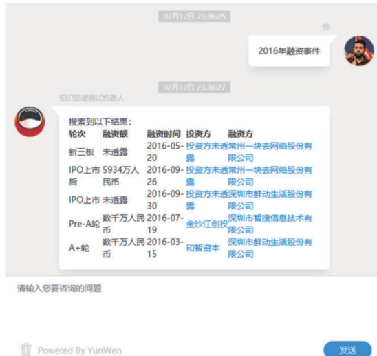
图 37 智能问答
